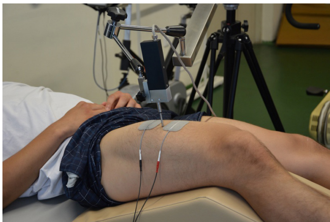
Слика 1 Начин постављања ТМГ електрода и сензора
